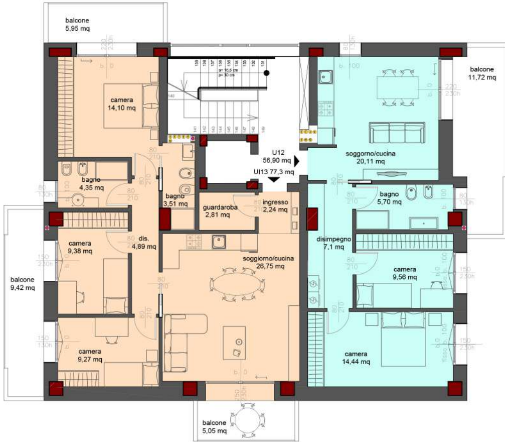
N PIANO 6° quota + 18.67 m
