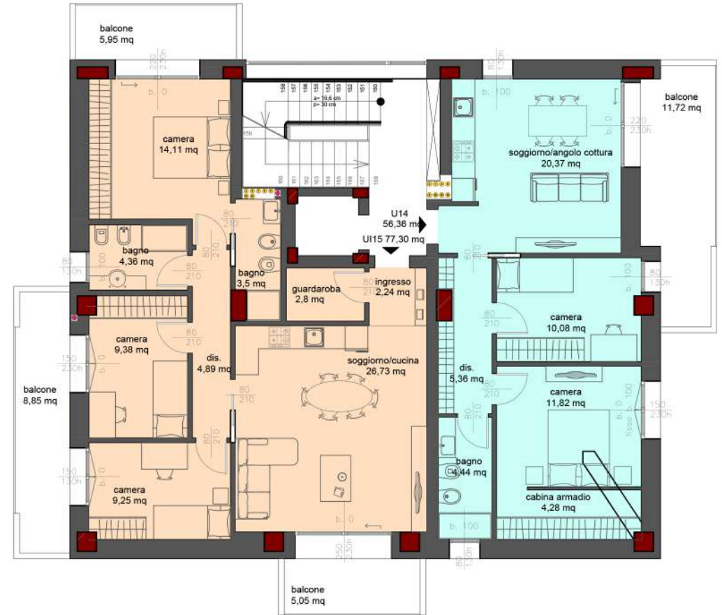
N PIANO 7° quota + 21.82 m
